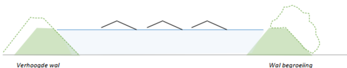
Principedoorsnede inpassing op waterbassins bij te lage omwalling
