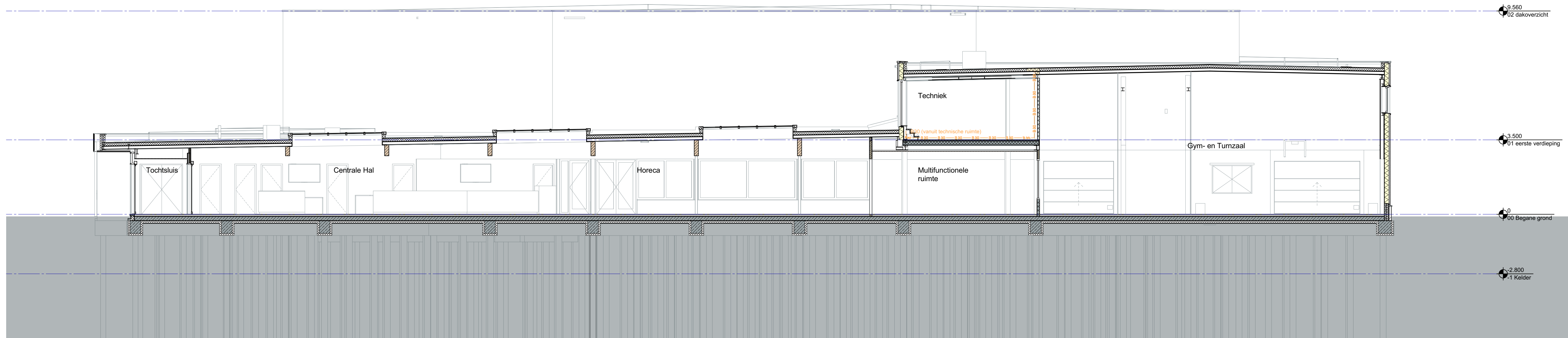
Doorsnede D-D
