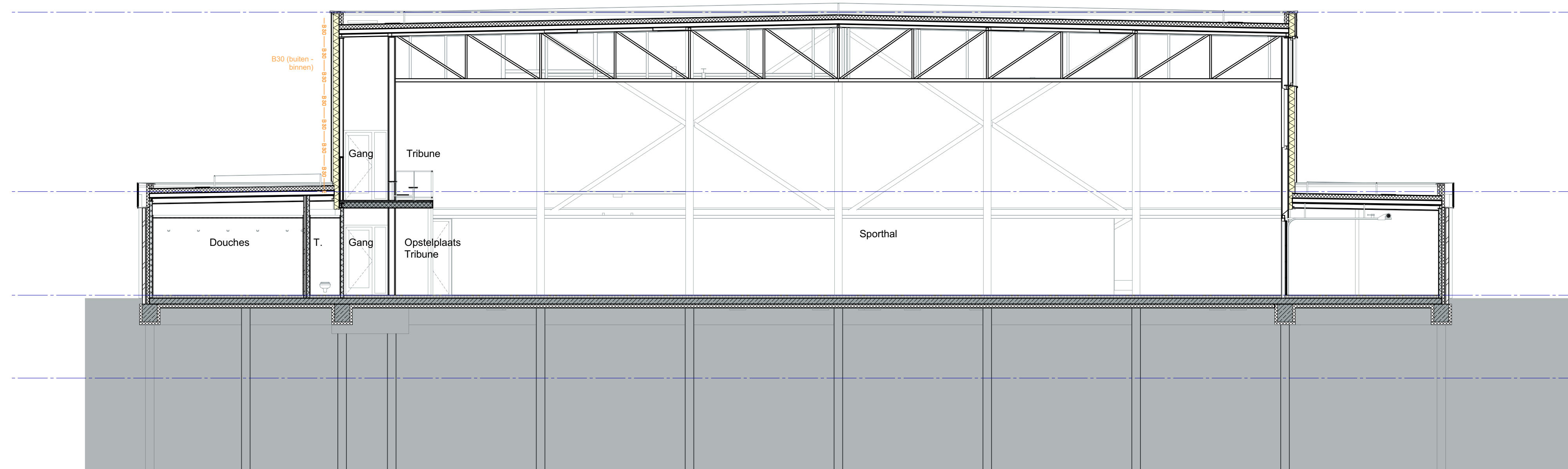
Doorsnede C-C
