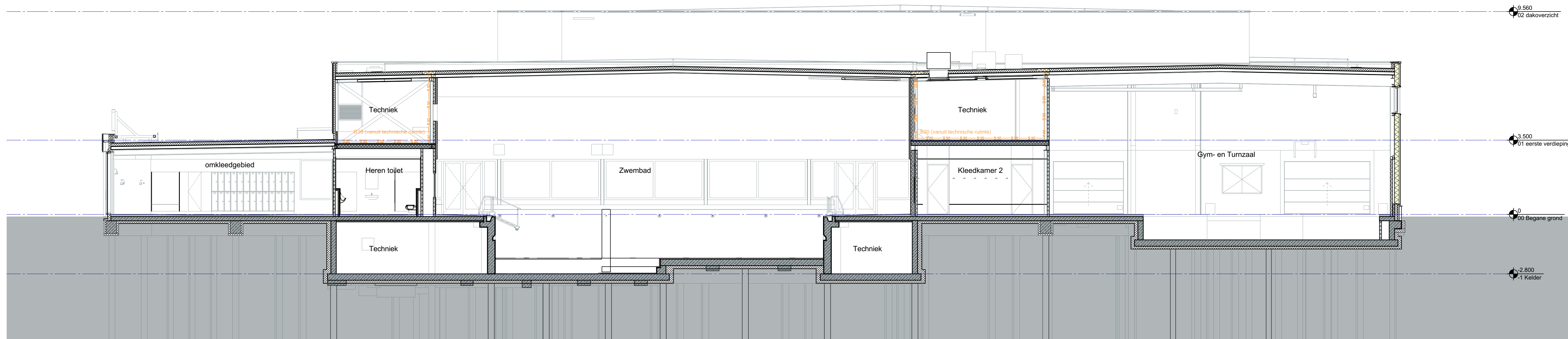
Doorsnede B-B
