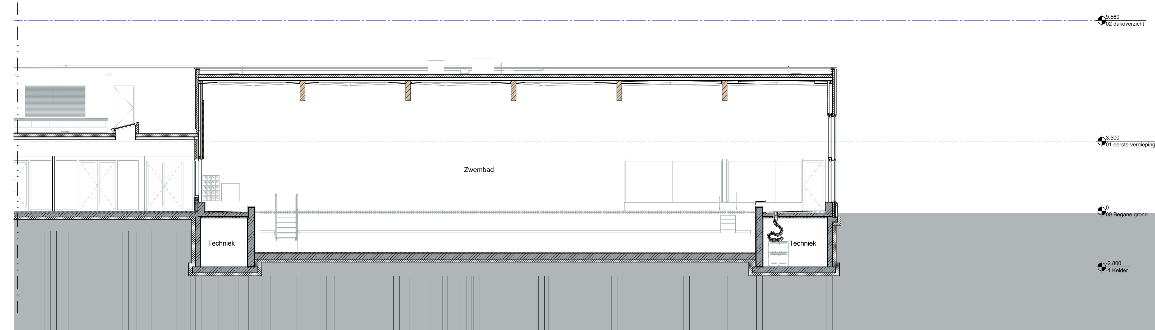
Doorsnede A2-A2
