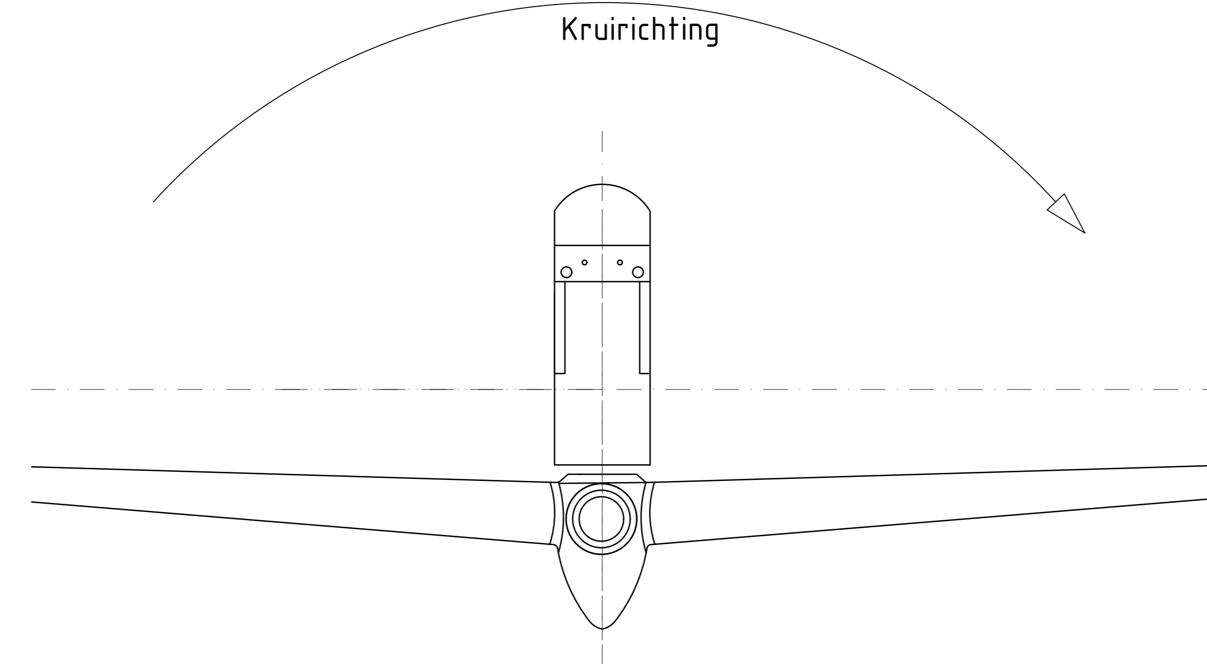
Bovenaanzicht Gondel
