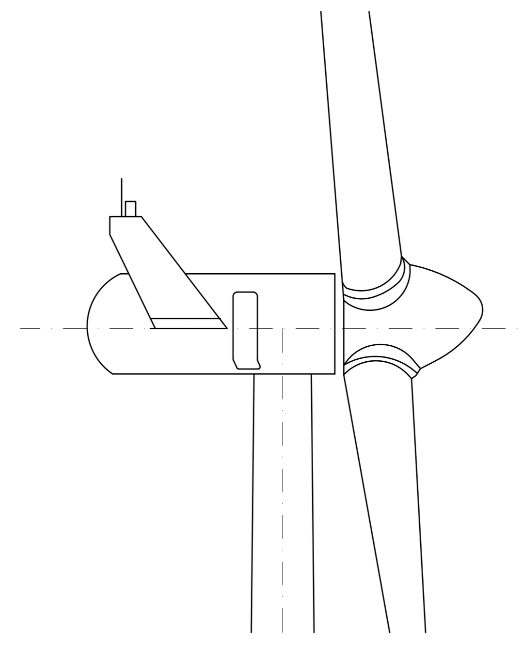
Zijaanzicht Gondel
